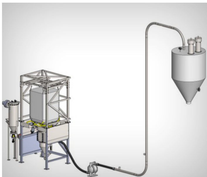
拆包站
